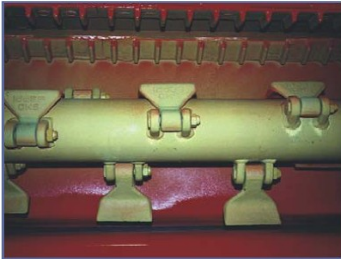
Tambur cu dispunere spirala a ciocanelor si contracutit forjat
