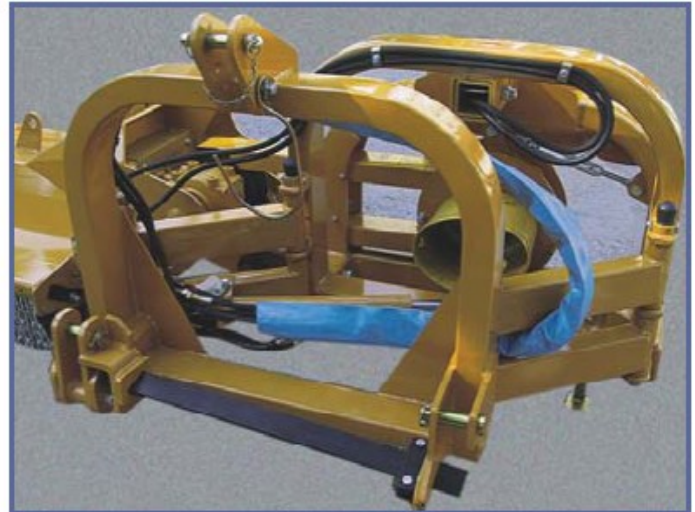
Optional: sistem de prindere in 3 puncte cu mecanism hidraulic de pozitionare laterala
